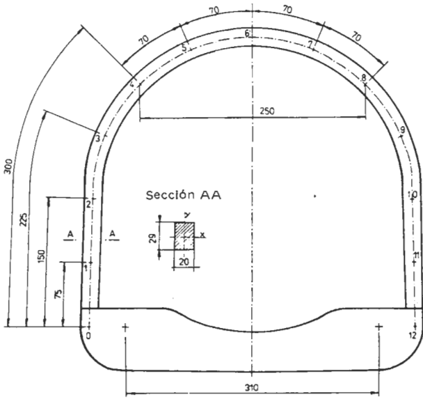
Fig. 3. Modelo de situación de las Secciones.
