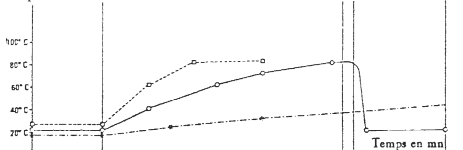
Temperatura - tiempos de secado en función del reactivo
